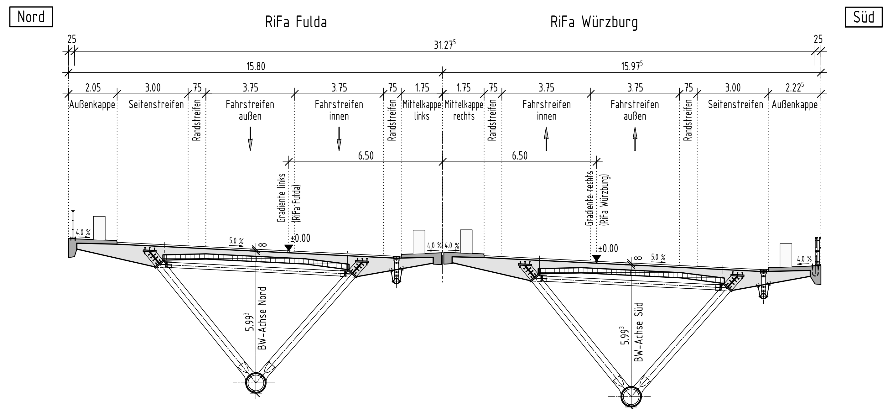
Regelquerschnitt M=1:100
