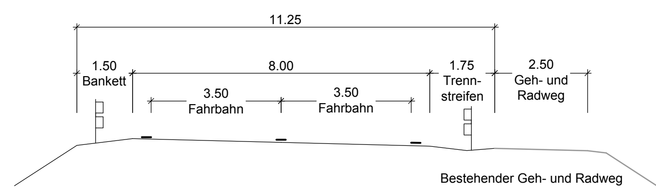
RQ Provisorium M 1:100
