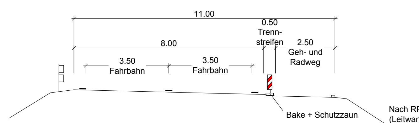
RQ Provisorium M 1:100
